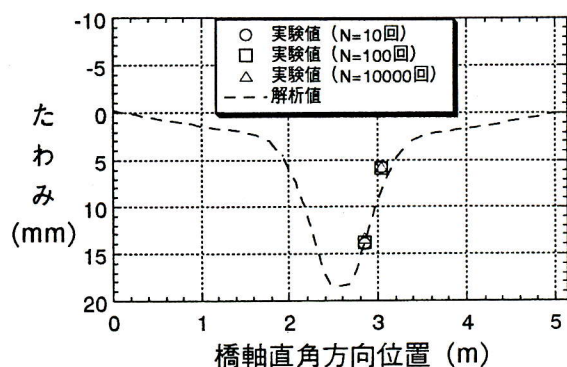
図4 デッキプレート鉛直たわみ分布
