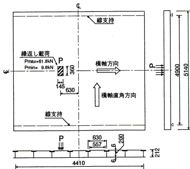
図2 供試体の形状
