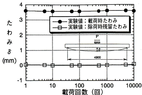
図3 床版下面鉛直たわみの履歴
