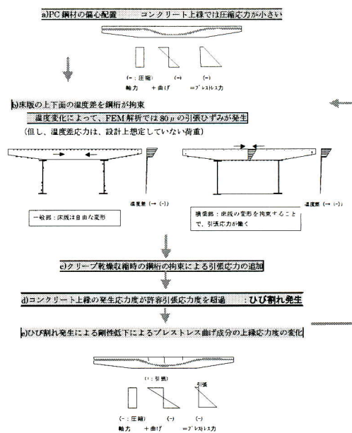
図-5 ひび割れ発生のフロー
