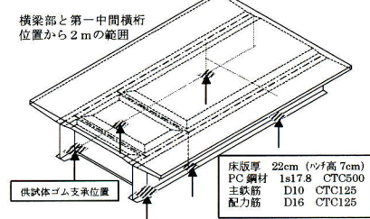
図-2 実験供試体のモデル化範囲
