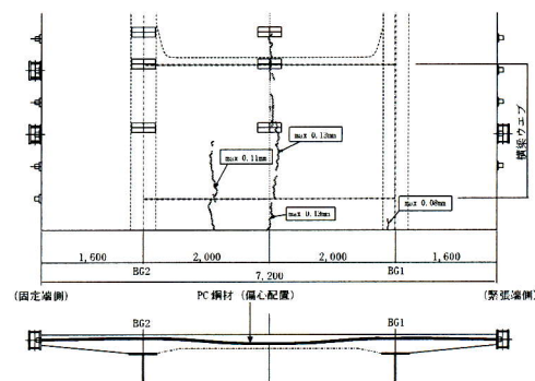
図-4 床版クラックマップ
